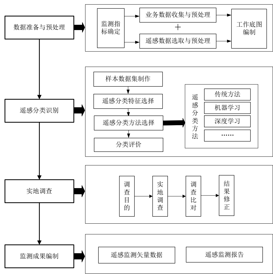
图 1 监测流程图
