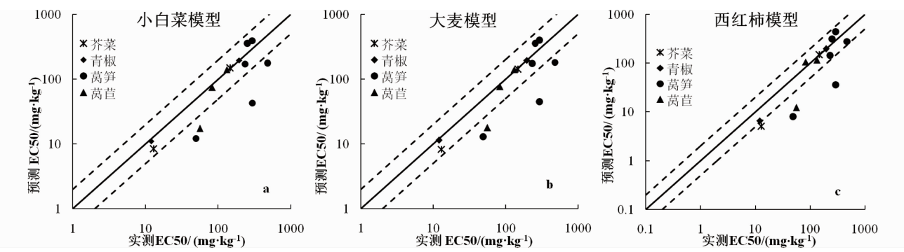
图 2 各物种镍 EC 50 测定值与预测值之间的相关性 注:实线代表 1: 1 的直线,虚线代表 2 倍的预测区间 Fig. 2 Correlation between the measured and predicted Ni EC 50 values for different species
