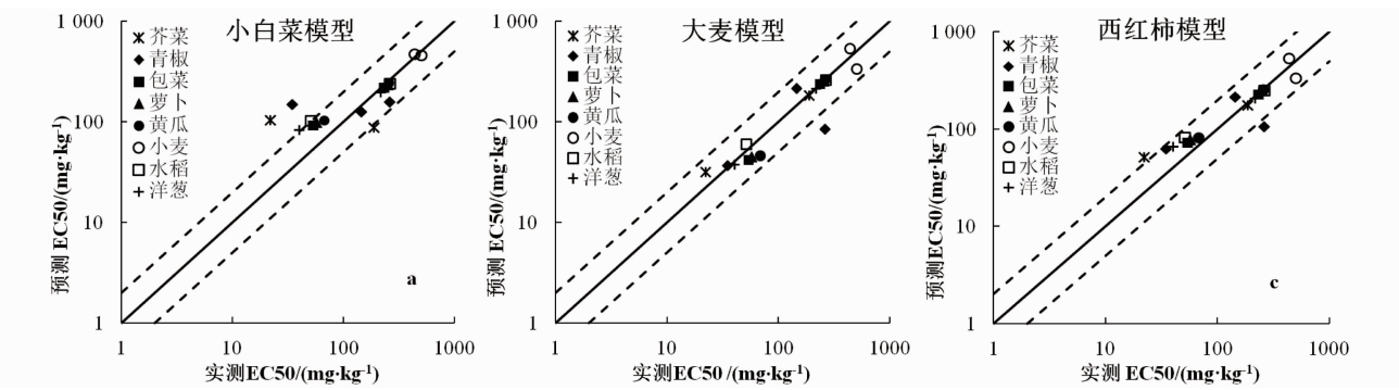
图 1 各物种铜 EC 50 测定值与预测值之间的相关性 注:实线代表 1: 1 的直线,虚线代表 2 倍的预测区间 Fig. 1 Correlation between the measured and predicted Cu EC 50 values for different species
